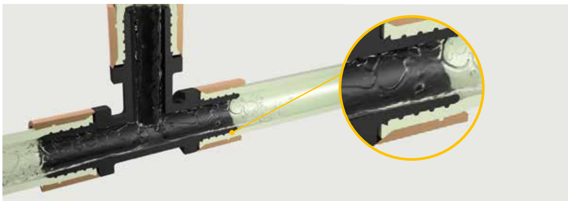
Push savienojuma šķērsgriezums
